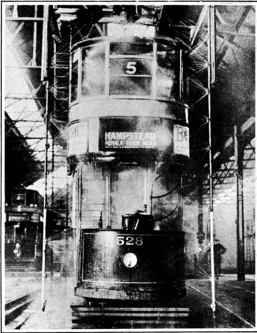
La instalación de este nuevo e ingenioso aparato para lavar tranvías, utilizado por una gran compañía londinense de transportes, ha sido de resultados tan eficaces, que ha podido suplir ventajosamente la labor de trescientos hombres... ¡El maquinismo se impone!
